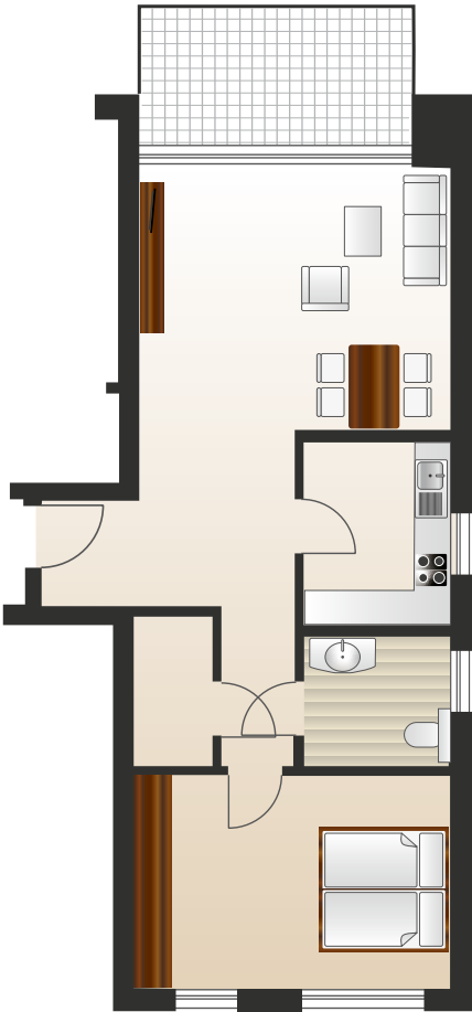
Wohnung 1.15 Gesamtwohnfläche: 73,74 m²
