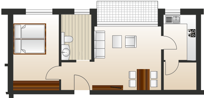
Wohnung 2.19 Gesamtwohnfläche: 56,38 m²
