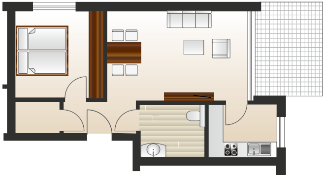
Wohnung 2.20 Gesamtwohnfläche: 56,82 m²
