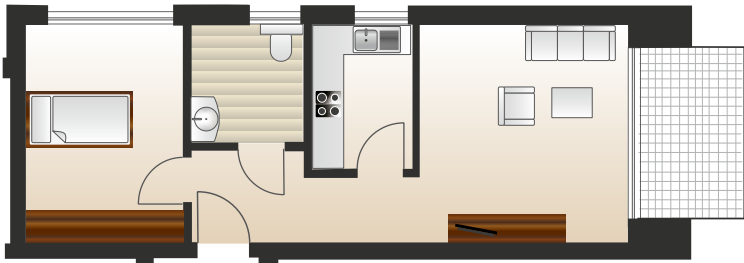
Wohnung E.26 Gesamtwohnfläche: 48,79 m²
