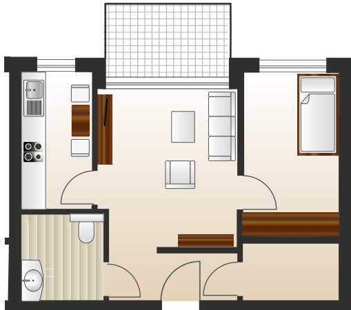
Wohnung 1.14 Gesamtwohnfläche: 48,51 m²
