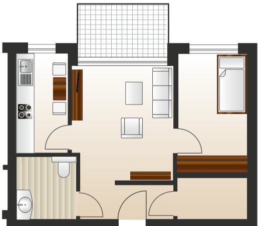
Wohnung 1.12 Gesamtwohnfläche: 48,51 m²
